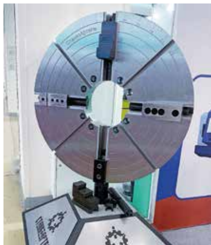
Рис. 2. Патрон \varnothing 1000 мм для станков 1Н65, 1М65, РТ117
