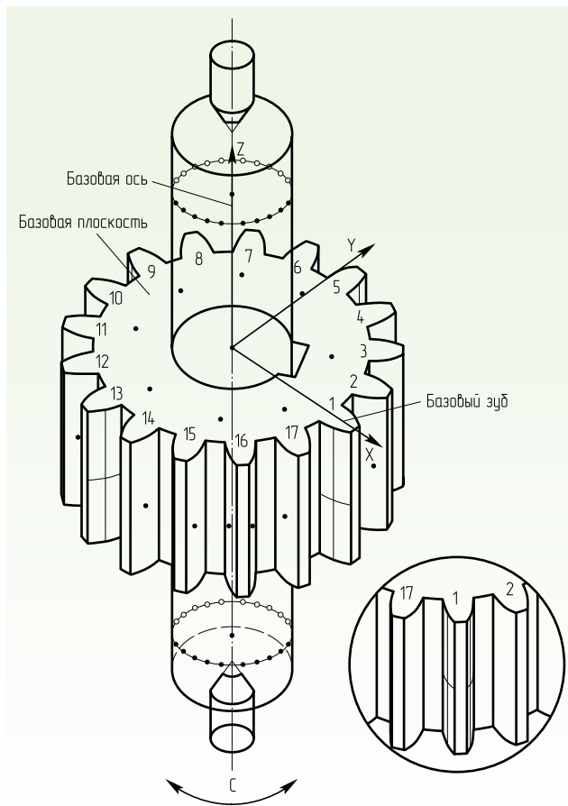
Рис. 5. Типовая стратегия четырехкоординатных измерений шестерни
