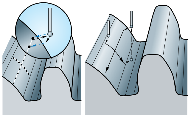
Рис. 6. Стратегии измерения боковых поверхностей зубьев
