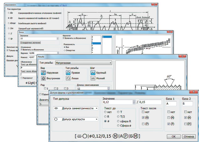
Рис. 10. Специализированные формы для редактирования технологических параметров
