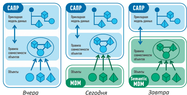
Рис. 7. Консолидации знаний о поведении и взаимодействии информационных объектов в семантической MDM-системе
