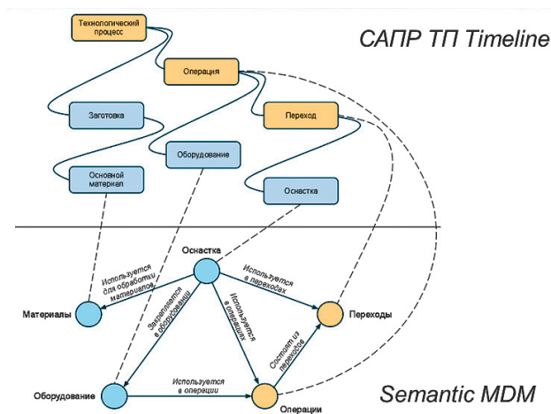
Рис. 8. Модель технологического процесса в САПР TP Timeline – это «тонкий клиент» семантической модели НСИ в Semantic MDM
