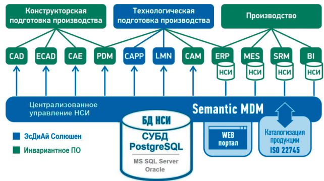
Рис. 15. Архитектура инженерного программного комплекса на платформе отечественной MDM-системы
