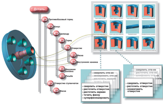
Рис. 5. Библиотека КТЭ, объединяющая интересы систем CAD и САПР ТП
