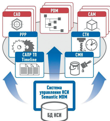
Рис. 14. Конструкторско-технологический программный комплекс на базе Semantic MDM
