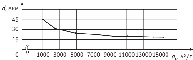
Рис. 2. Зависимость диаметра частиц от суммарного ускорения
